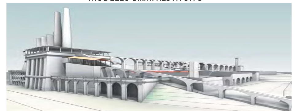
MODELLO B.I.M. RESTITUITO
